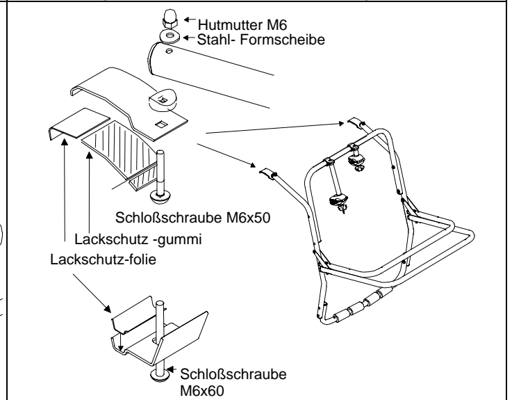
6. Bekleben Sie die oberen und die unteren Einhängeteile mit den Schutzfolien bzw. Schutzgummis. Evtl. sind die Schutzgummis mit einer Schere zu kürzen. Verschrauben Sie die oberen Einhängeteile an den Trägerholmen.
